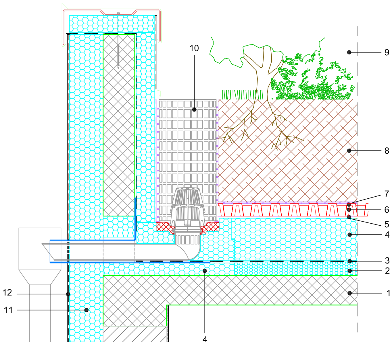
SASTAV SISTEMSKOG RJEŠENJA (dimenzije uskalditi s proračunom građevne fizike):
